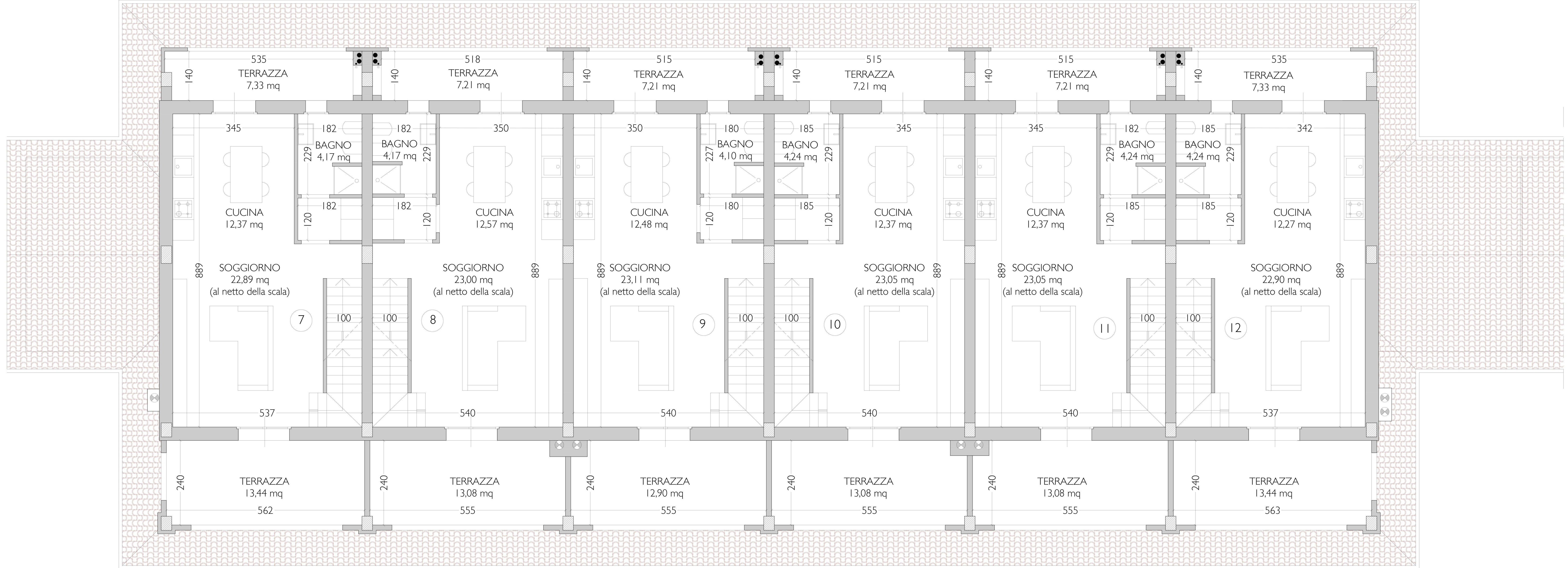
PIANTA PIANO PRIMO
