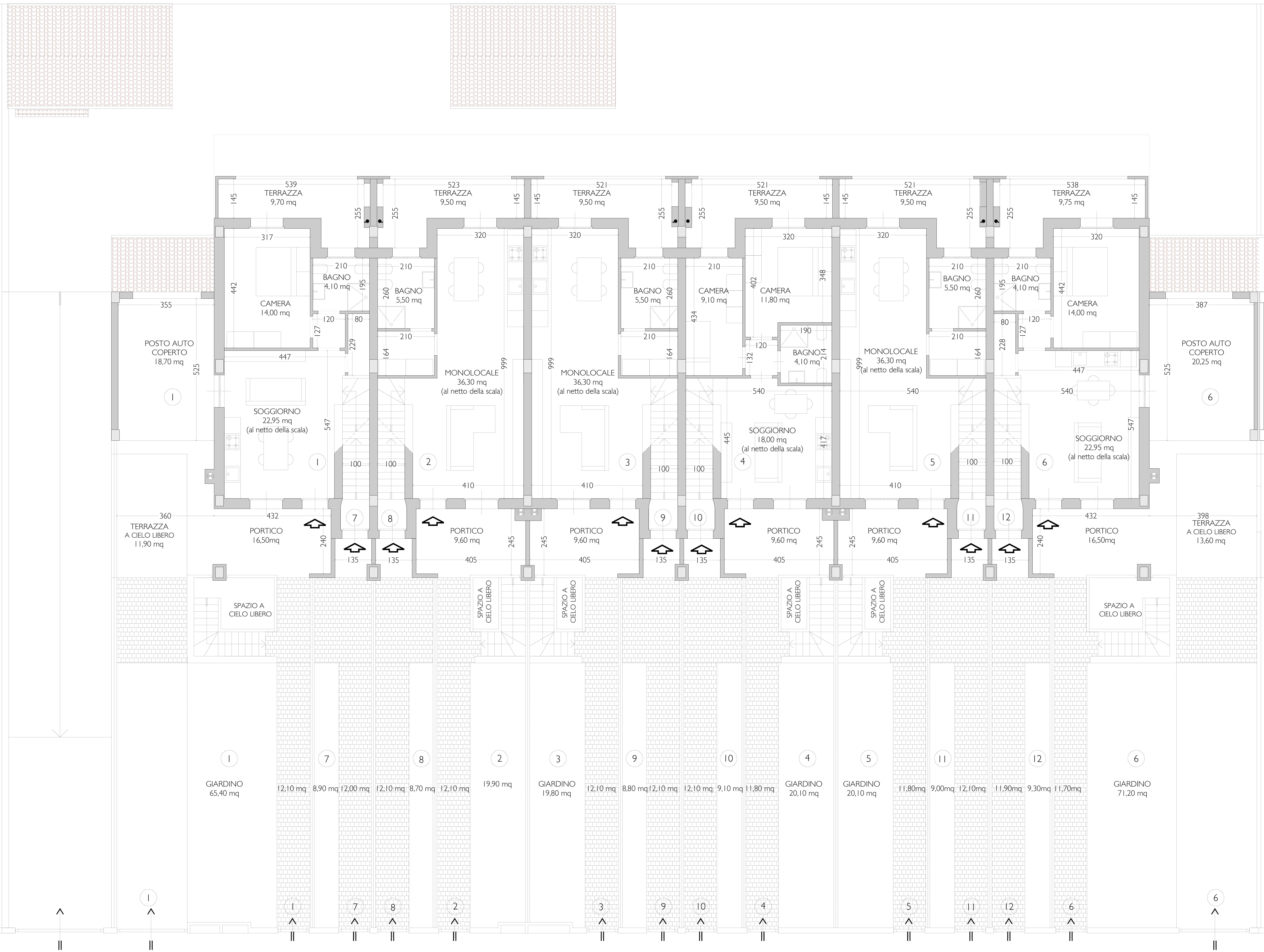
PIANTA PIANO TERRA
